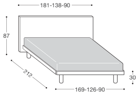
LM40Q Base QUADRA
