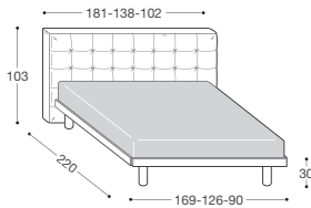
LM12Q Base QUADRA
