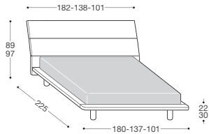
LM7K Base ORIZZONTE
