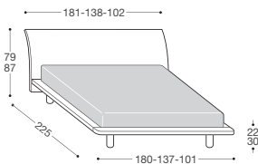
LM1K Base ORIZZONTE
