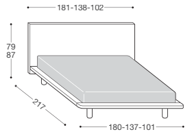
LM40K Base ORIZZONTE
