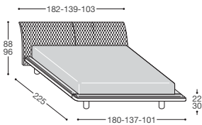
LM19E Base ERGO
